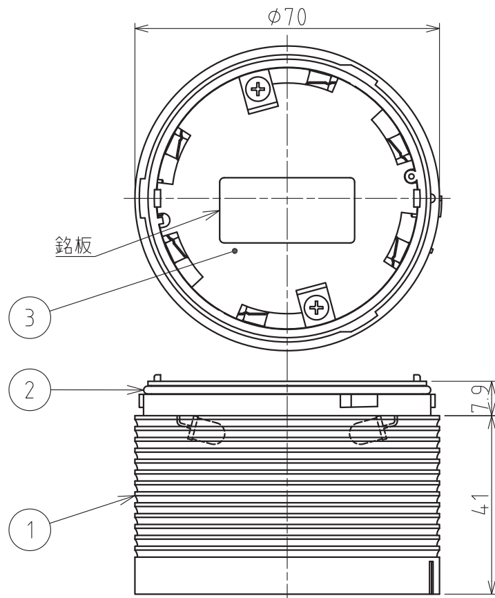
外観寸法図
