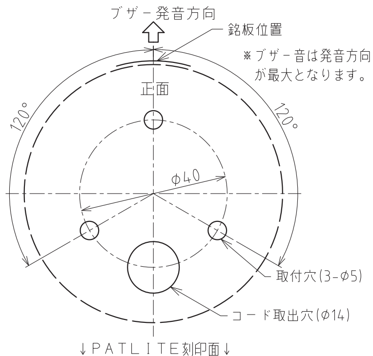
取付面寸法図 (1:1)
