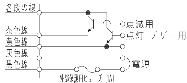
オープンコレクタ (NPN型トランジスタのみ)
