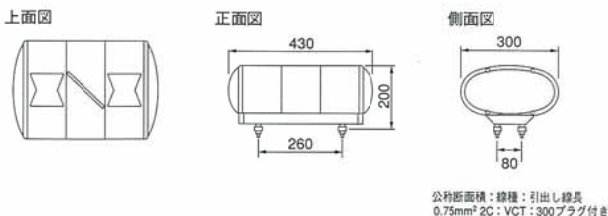
外観図 (mm)
