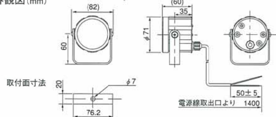
外観図 (mm)
