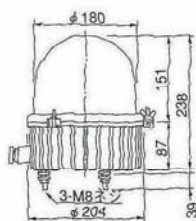
外観図(mm)
