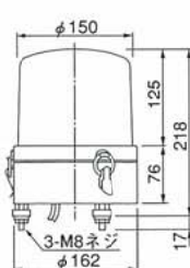
外観図(mm)
