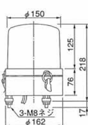
外観図(mm)
