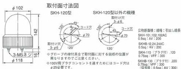
外観図(mm)
