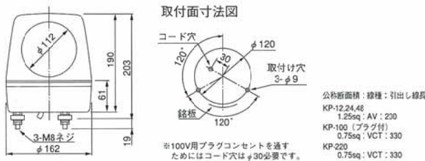
外観図(mm)
