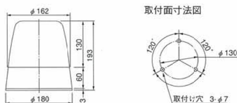
外観図(mm)
