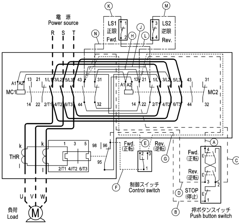
(1) RMUF300、RMUF400 三相回路
