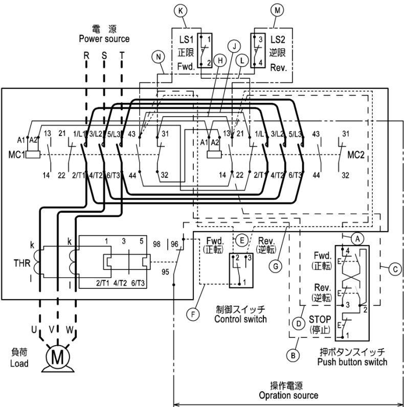
(2) RMUF300、RMUF400 独立電源回路
