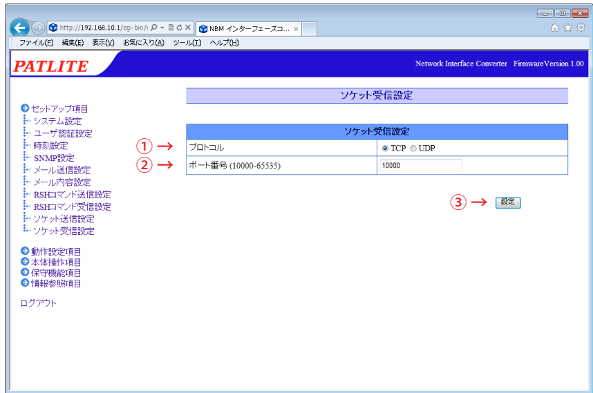
図 4.10.0-1 ソケット受信設定画面
