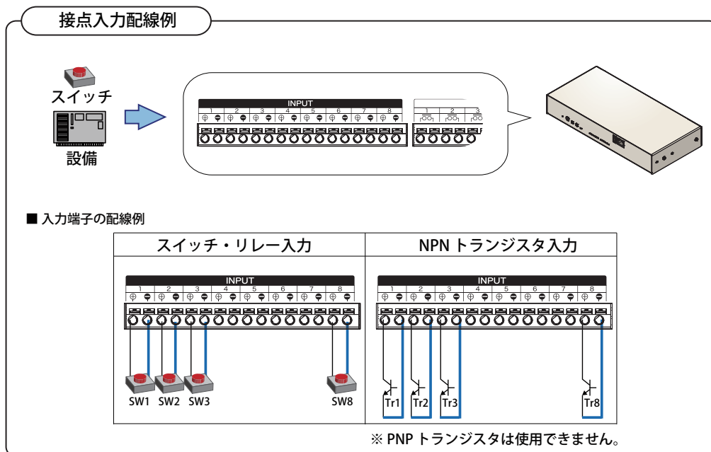
図 3.1.1-1 デジタル入力の接続例
