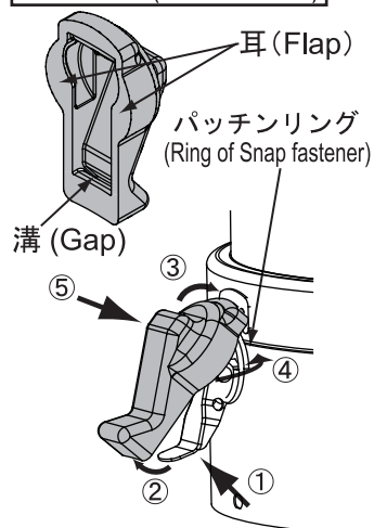
ゴムカバー (Rubber cover)
